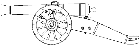
40.45.009 belegeringsaffuit en voorwagen
